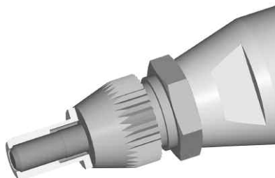
Figura 9 – Regolazione della posizione del cono
