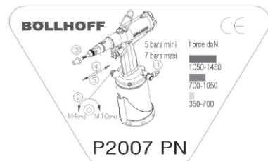
Abbildung 11 - Einstellhilfe
