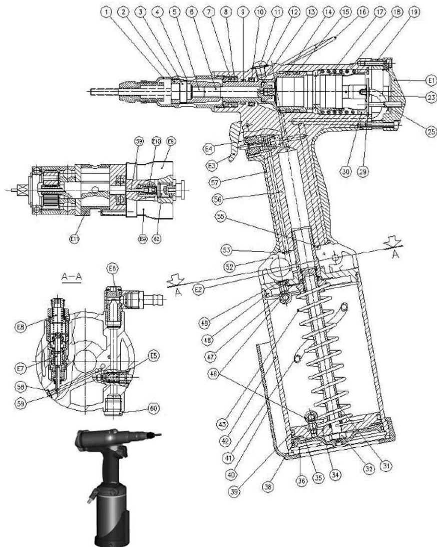
Abbildung 16 - Ersatzteileübersicht
